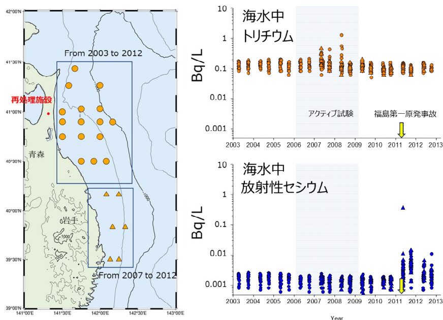
図 1 (左) 東日本北太平洋側沿岸海域での調査地点 (右) 海水中の放射性核種濃度。Shirovani et al. (2021, https://doi.org/10.1016/j.fusengdes.2021.112738 ) のデータから図を改編。
