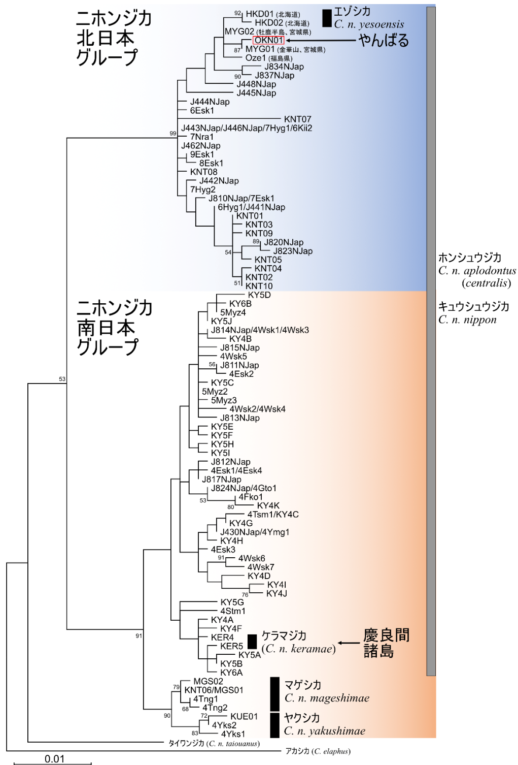
図2. ニホンジカのミトコンドリア DNA コントロール領域の分子系統樹。スケールバー (0.01 と書かれた横棒) は遺伝距離 (短いほど遺伝的に近く、長いほど遺伝的に遠い) を表し、ブートストラップ値が 50% 以上の分岐点にはその数値を示し、数値が大きいほどその枝が統計的に確からしいことを示している (作成、高木俊人)。
