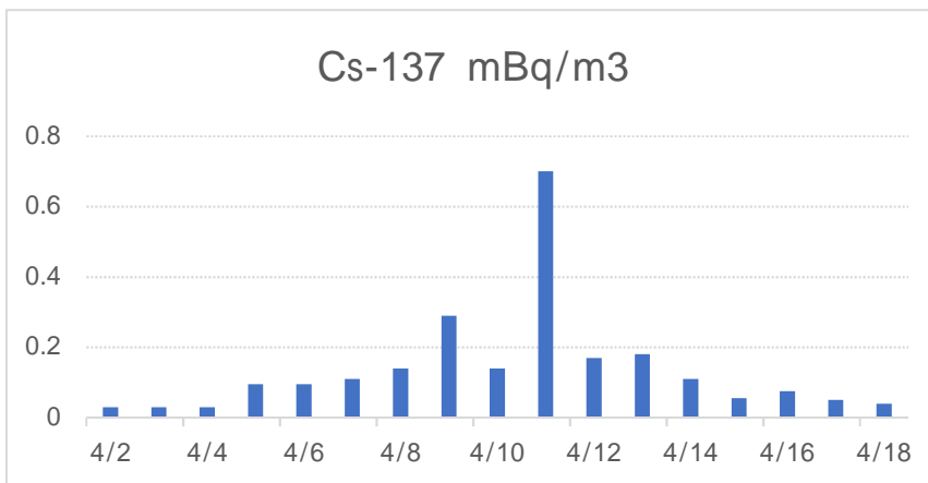
図2 2020年4月以降のキエフ市内における大気中放射性セシウム濃度の推移（データ提供：ウクライナ中央地球物理学研究所 レオナルド・タバチネ博士）
