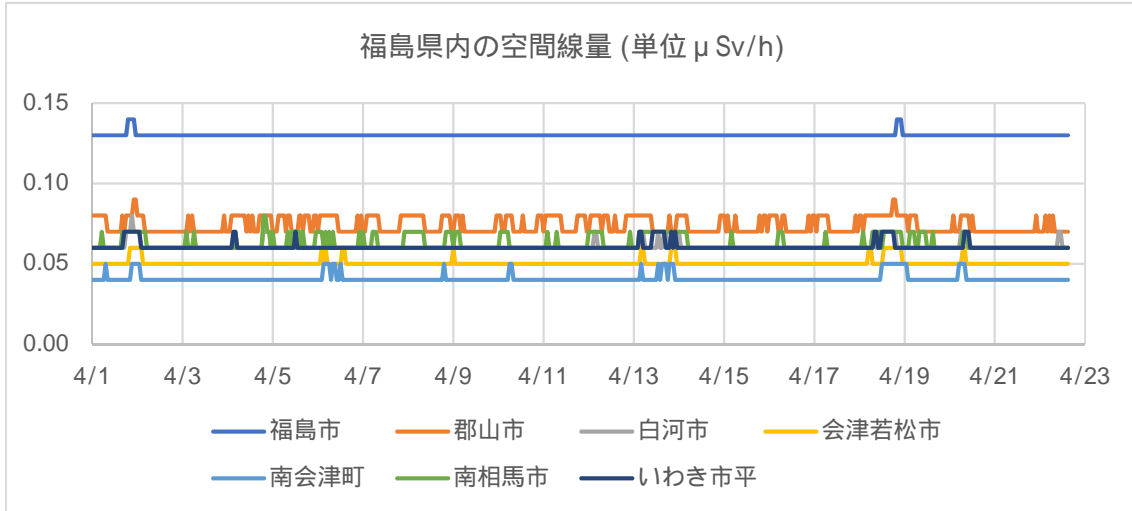
図4 福島県における2020/4/1から4/22 15:00までの空間線量のモニタリング結果
