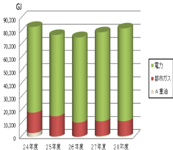
金谷川団地総エネルギー投入量の推移
