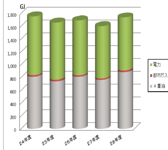
附属特別支援校総エネルギー投入量の推移
