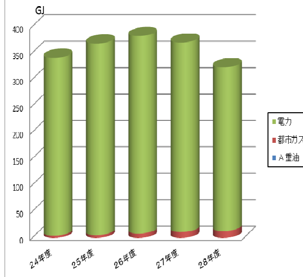
舟場町団地総エネルギー投入量の推移
