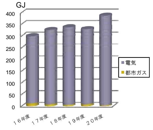
舟場町団地総エネルギー投入量の推移
